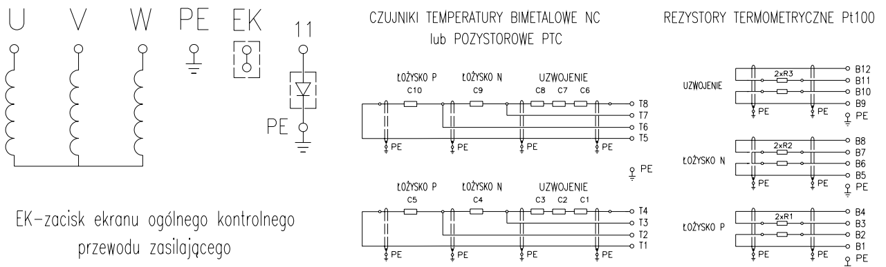
Rys.1 Schemat połączeń silnika
