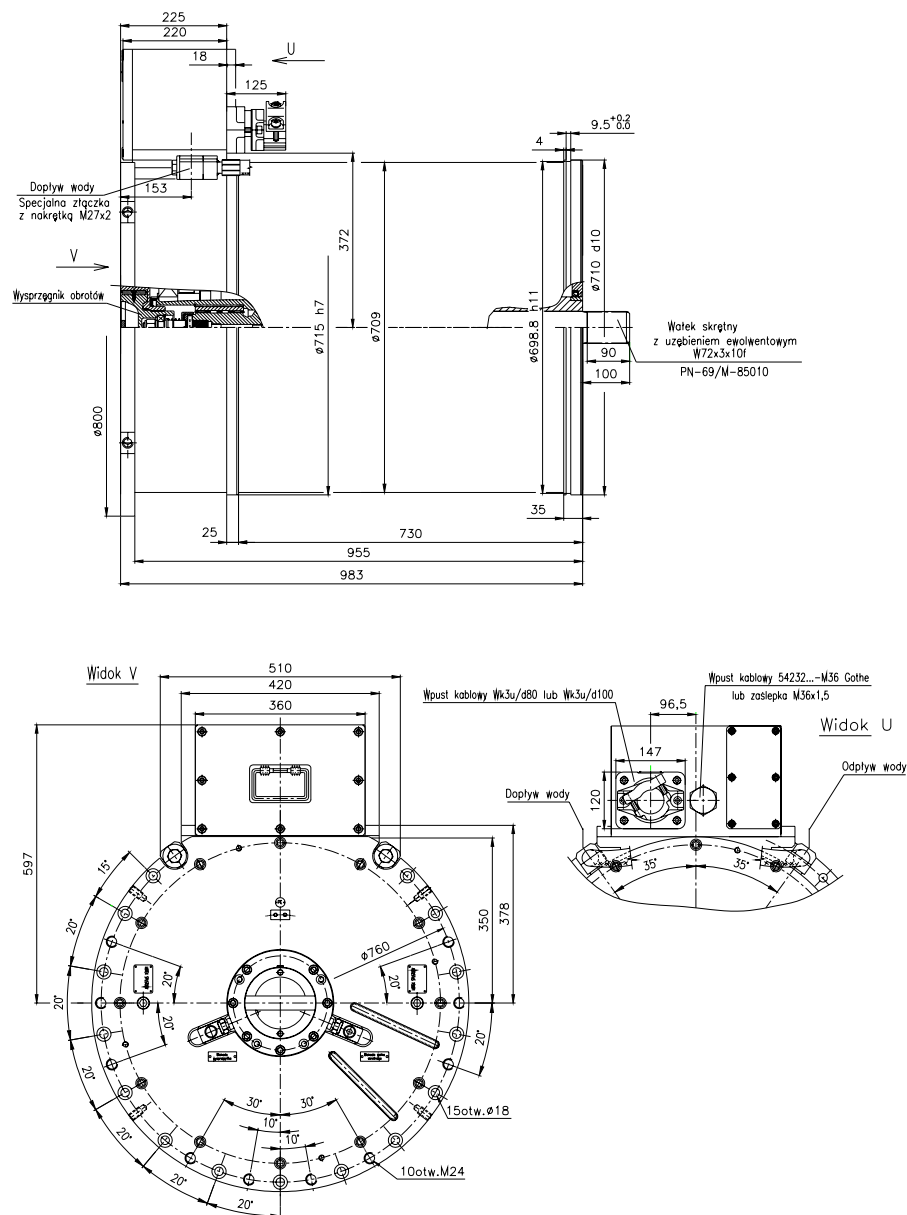
Rys.3 Wymiary montażowe i gabarytowe
