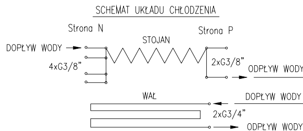
Rys.2 Schemat układu chłodzenia
