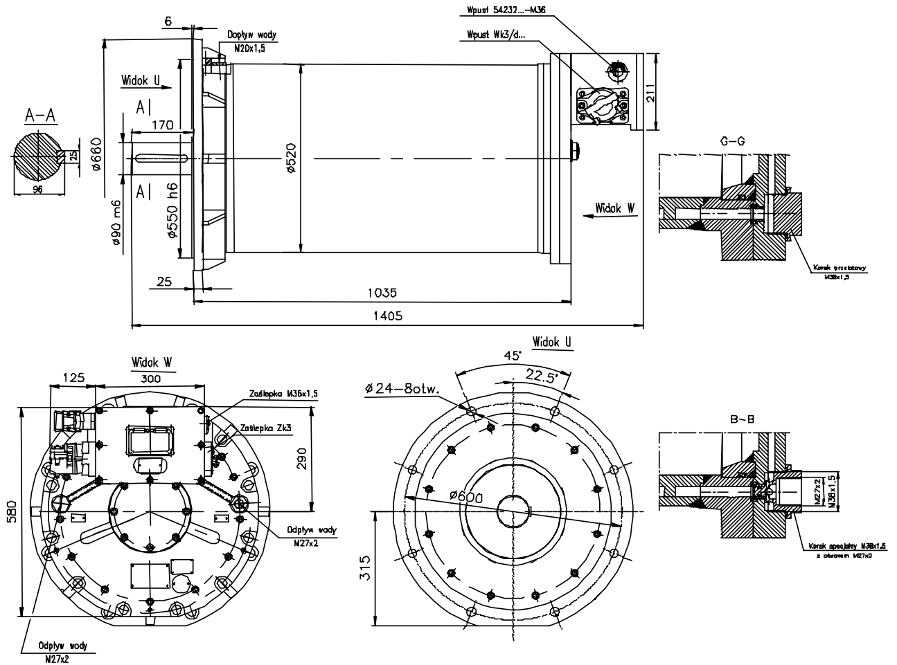
Rys.3 Wymiary montażowe i gabarytowe
